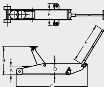
2T-C BOGIE PU 2T-C monteret med bogie system med polyurethan ruller.
