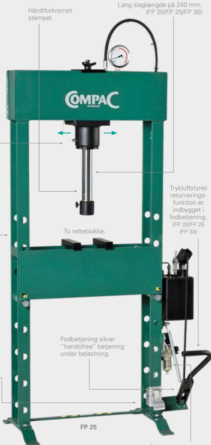
Lufttilslutning monteret med vandudskiller. (FP 20/FP 25/FP 30)
